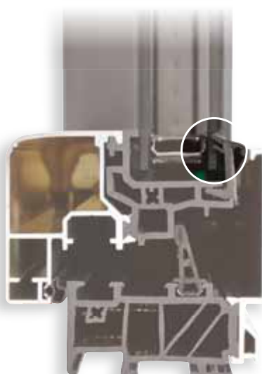
VITRAGE COLLÉ CE PROCÉDÉ DE FABRICATION REND L'ACCÈS PAR L'EXTÉRIEUR TRÈS DIFFICILE EN CAS DE TENTATIVE D'INTRUSION
